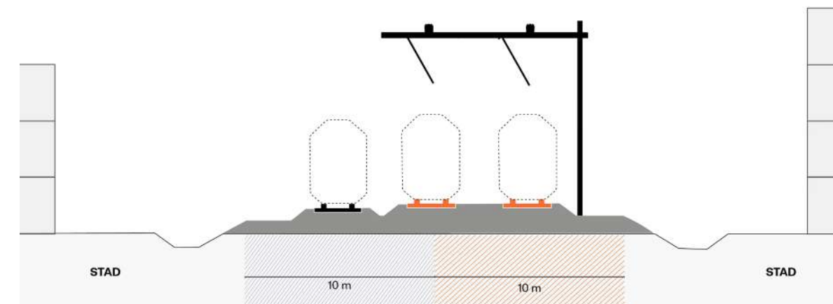
Principe uitgangssituatie 2 sporen naast bestaand spoor incl. bovenleiding
