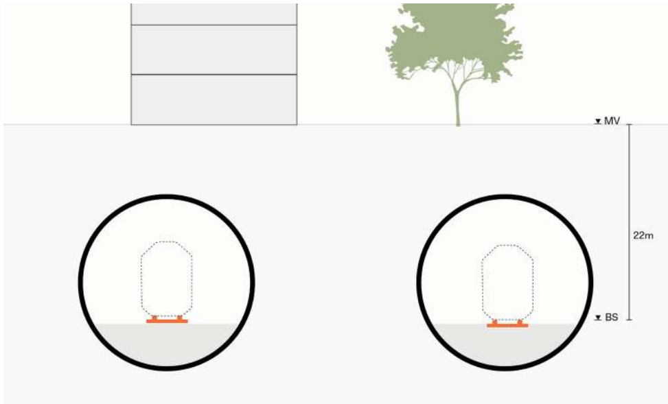
Principe uitgangssituatie 2 sporen in boortunnel
