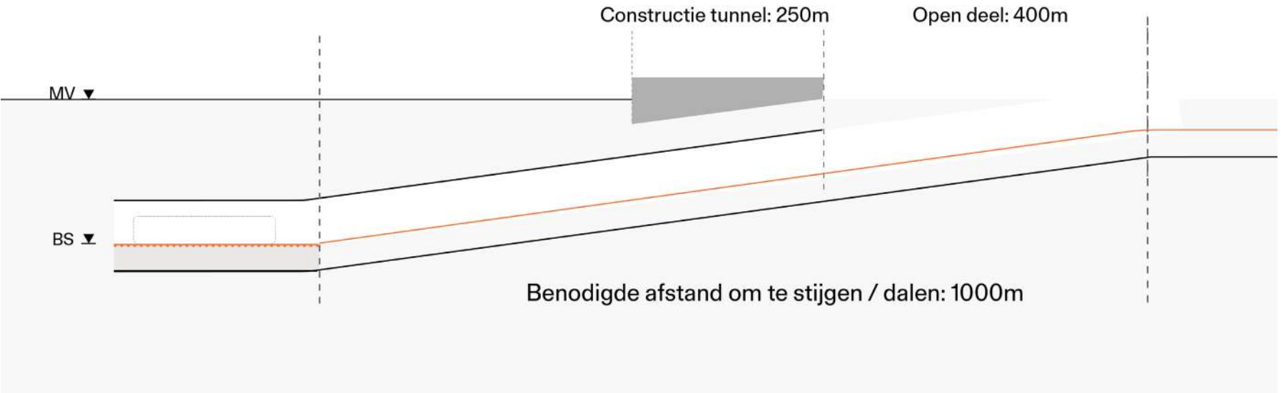
Principe uitgangssituatie 2 sporen in boortunnel naar maaiveld
