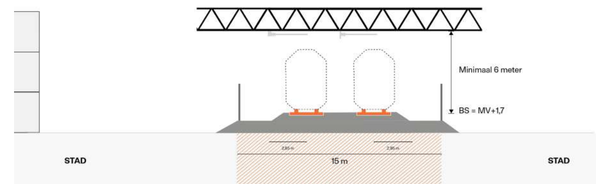
Principe uitgangssituatie 2 sporen incl. bovenleiding onder constructie
