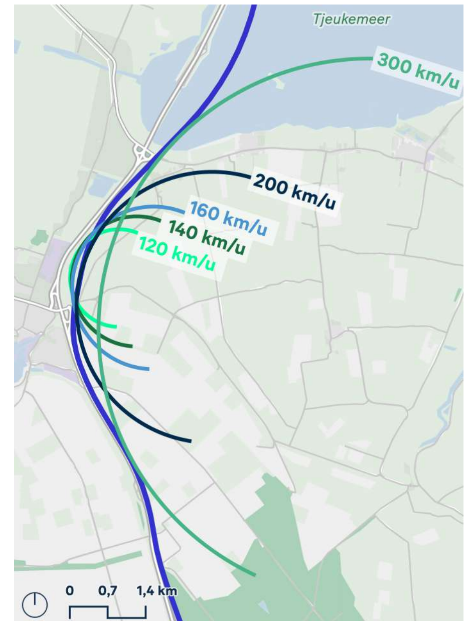
Voorbeeld benodigde boogstralen voor verschillende snelheden, geprojecteerd op het bundelingstracé bij Lemmer, zoals in onderzoek Lelylijn-alternatieven.
